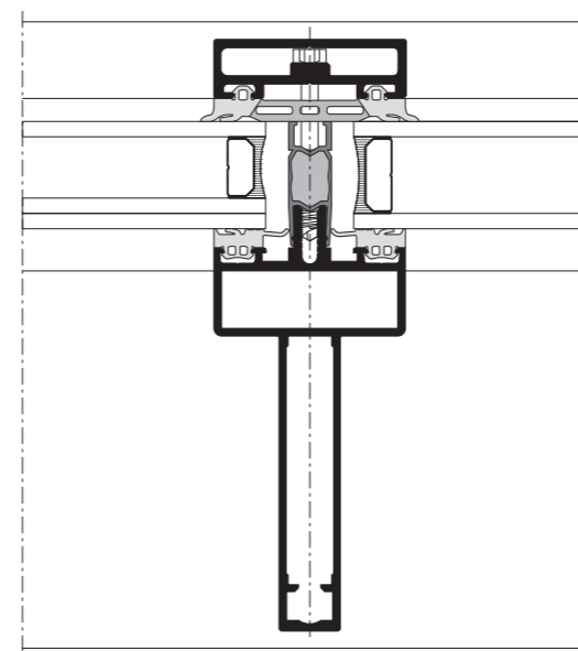
heroal C 50 ID sezione montante con listello pressore avvitato (sagoma stile acciaio)
