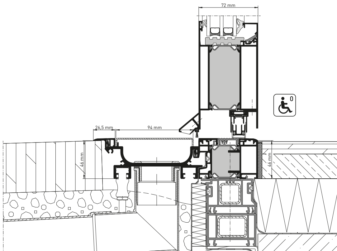
heroal D 72 s heroal DS, řez
