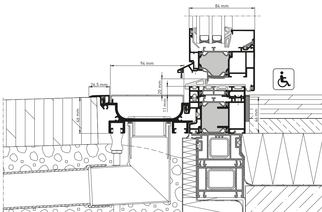
heroal W 72 s heroal DS, řez
