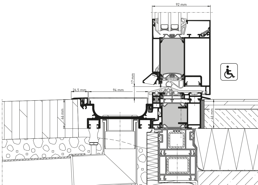
heroal D 92 UD s heroal DS, řez
