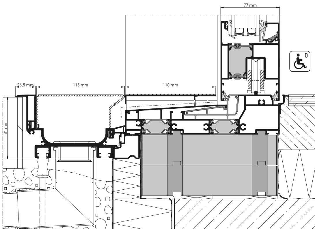
heroal S 77 SL s heroal DS, bezbariérové podle DIN 18040, řez
