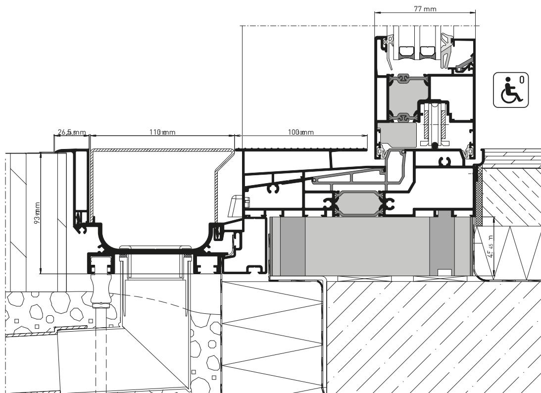
heroal S 77 s heroal DS, bezbariérové podle DIN 18040, řez
