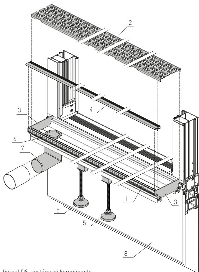
heroal DS, systémové komponenty
