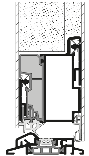
Zwischengeschraubte Schwelle mit flächenbündigen Flügel
