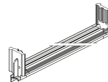
Neue Türabschlussdichtung mit eckvulkanisierter Formecke für Flügel flächenbündig
