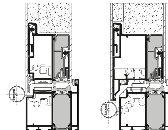
heroal D 72 PF EM bs, Schnittdarstellungen
