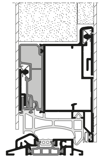
Zwischengeschraubte Schwelle mit aufschlagendem Flügel
