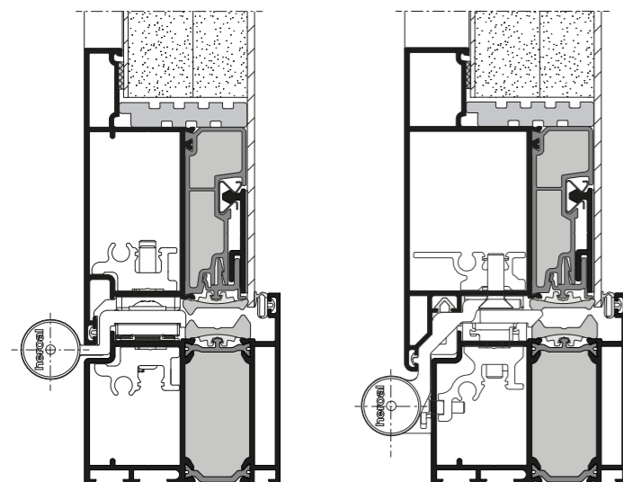
heroal D 72 PF EM es, Schnittdarstellungen
