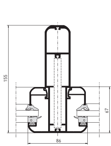
Krokve pro velká zatížení střechy
