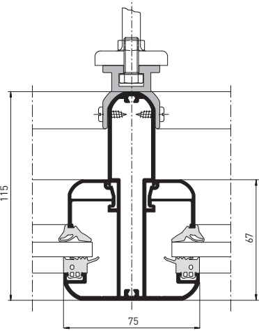
Profil krokve s držákem na protisluneční ochranu
