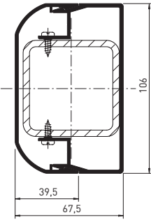
Obložení překladu
