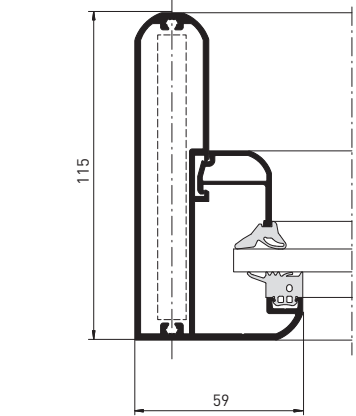
Řez krokví a koncovou krokví
