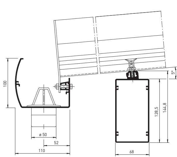
Přesah střechy u upevnění podpěr
