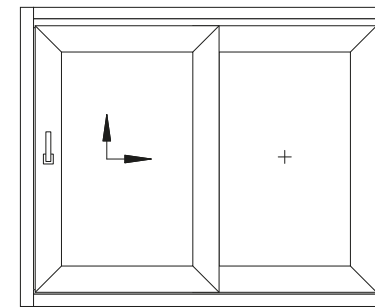
Eén bewegende vleugel, die naar links opent
