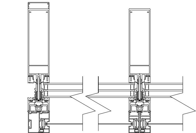
Profilé de champ d'extrémité et de champ central
