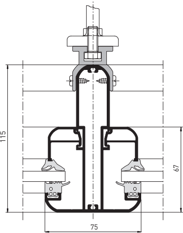
Profil de chevrons avec un support pour protection solaire
