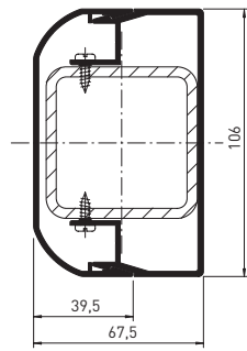
Revêtement du linteau
