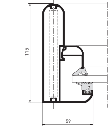
Coupe des chevrons et chevrons d'extrémité
