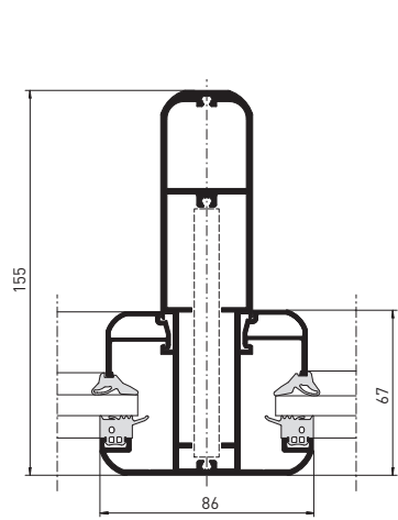
Chevrons pour les charges de toit élevées
