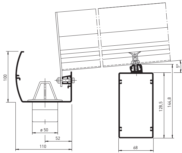
Avancée de toit fixation des supports
