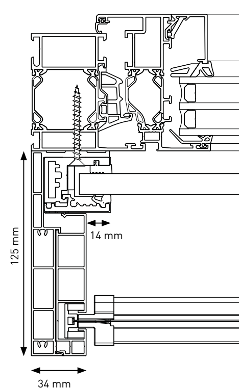
heroal VS Z plus auf heroal W 72 Aluminiumfenster
